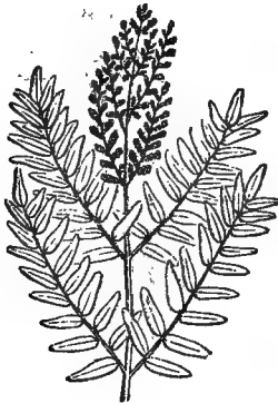
OSMUNDA REGALIS. (Royal Fern.)
